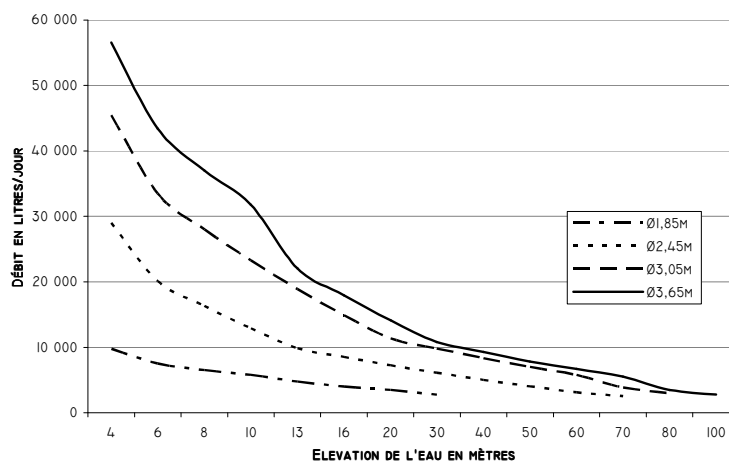
DÉBIT EFFECTIF POUR LES 4 DIFFÉRENTS DIAMÈTRES DE ROTOR*
